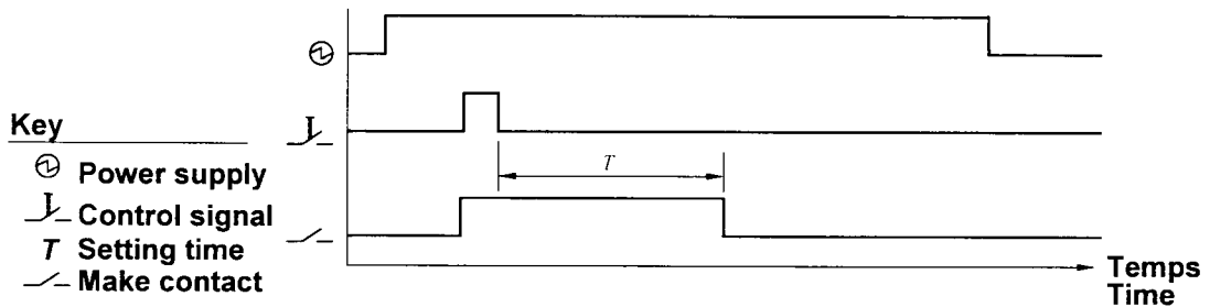
图3 有控制信号的释放延时继电器
