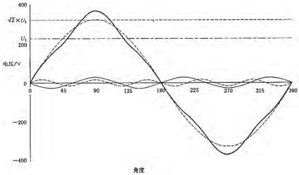
图 7 尖顶波波形
