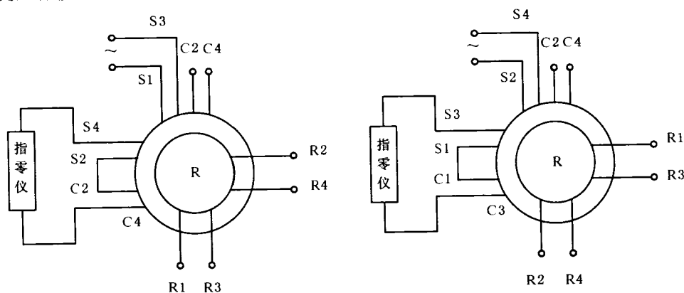
图 19 补偿绕组交轴电压试验路线
