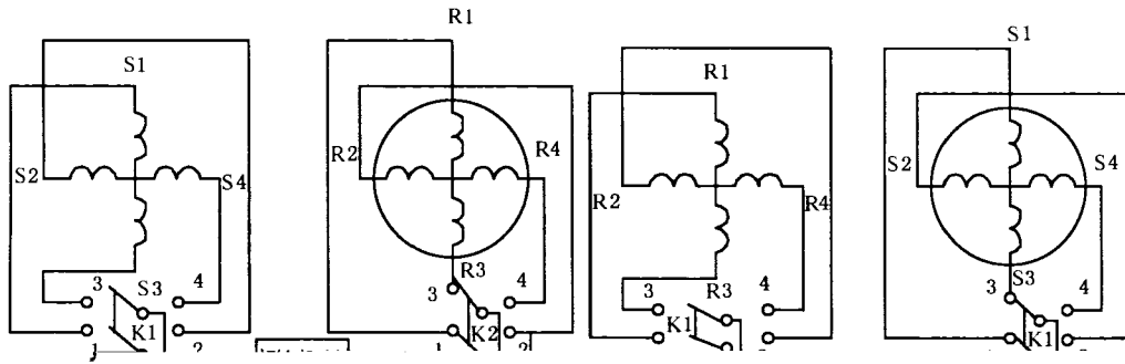
图 9 相敏电压表方向校正线路图
