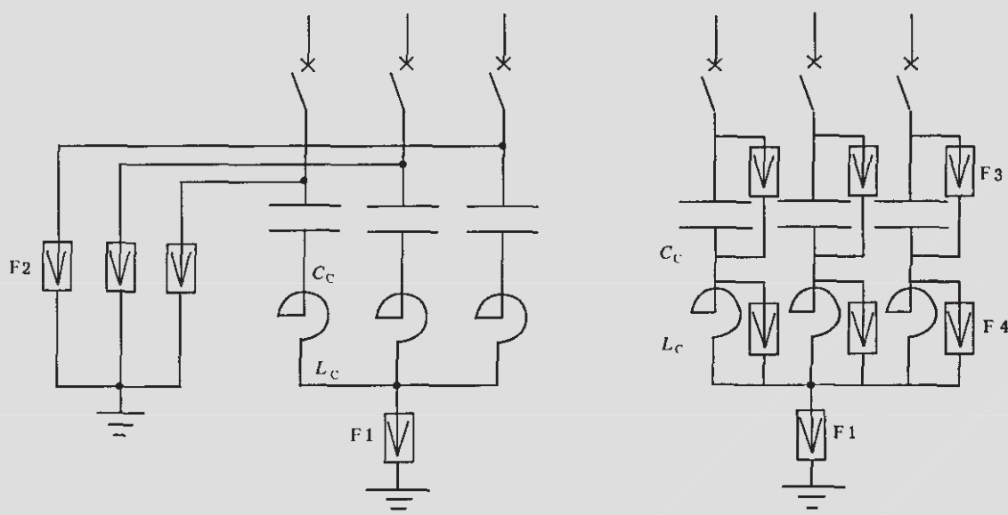
a) 单相重击穿过电压的保护接线
